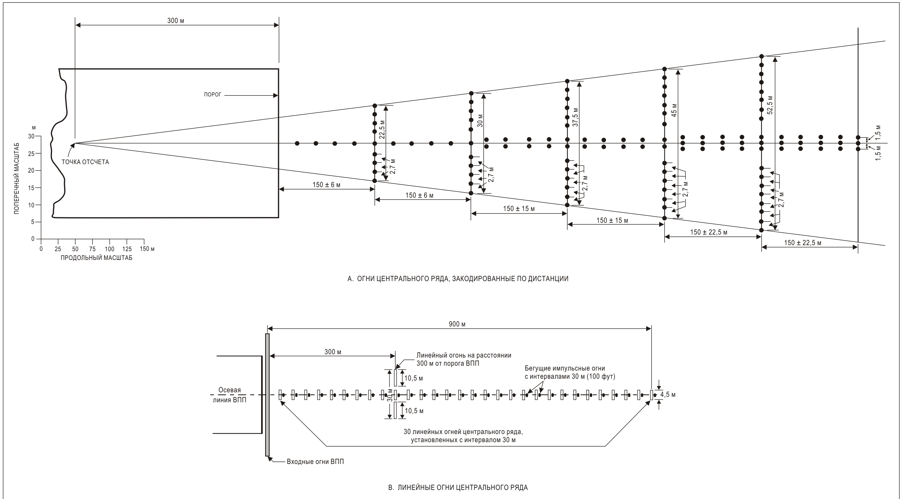
Рис. А-7. Системы огней приближения для точного захода на посадку по категории I
