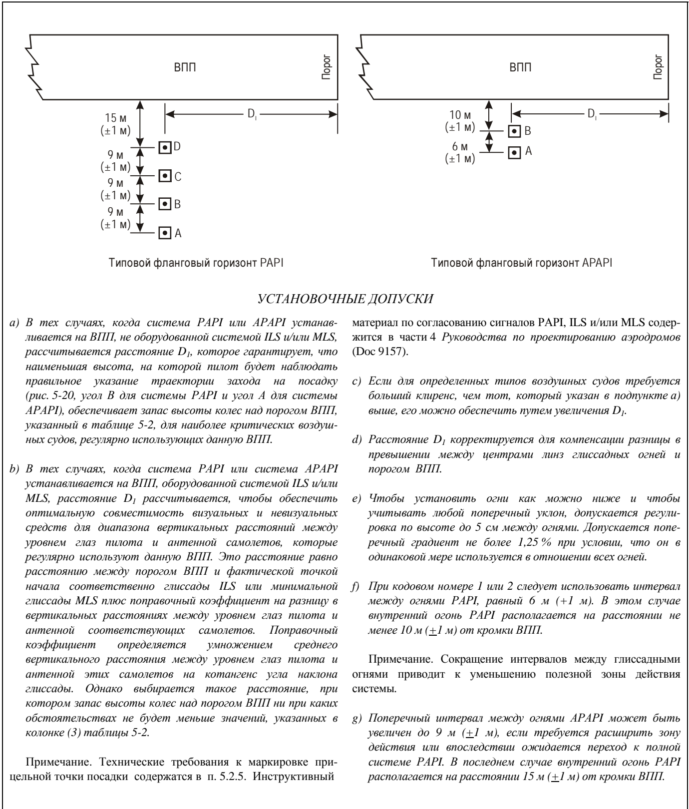
Рис. 5-19. Расположение PAPI и APAPI
