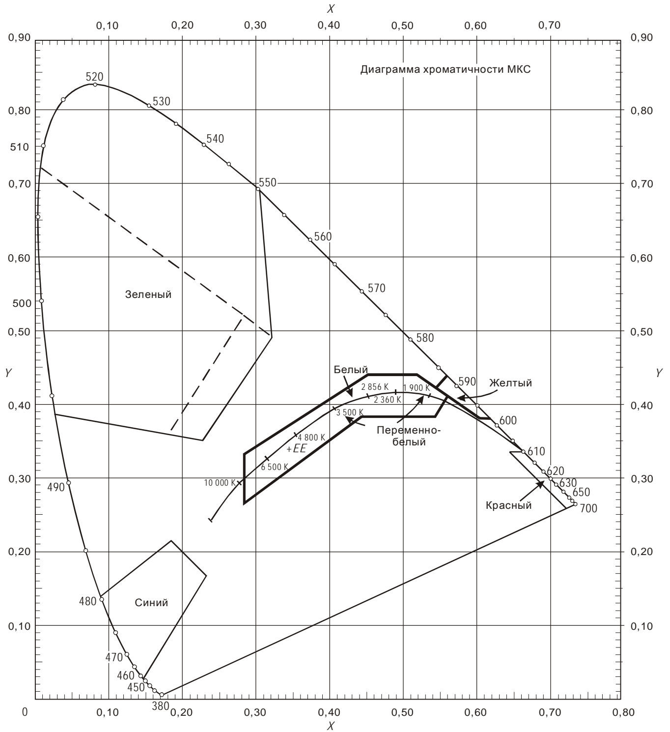
Рис. А1-1. Цвета аэронавигационных наземных огней
