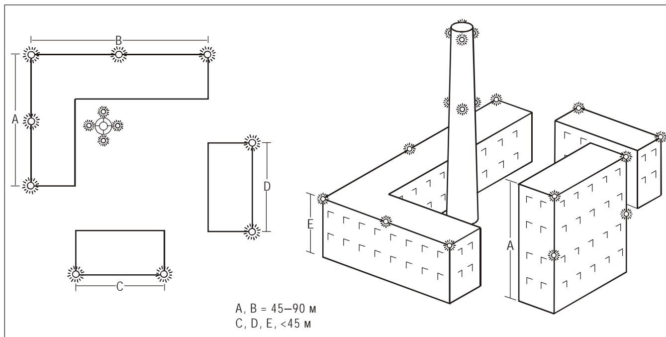
Рис. 6-3. Световое ограждение зданий
