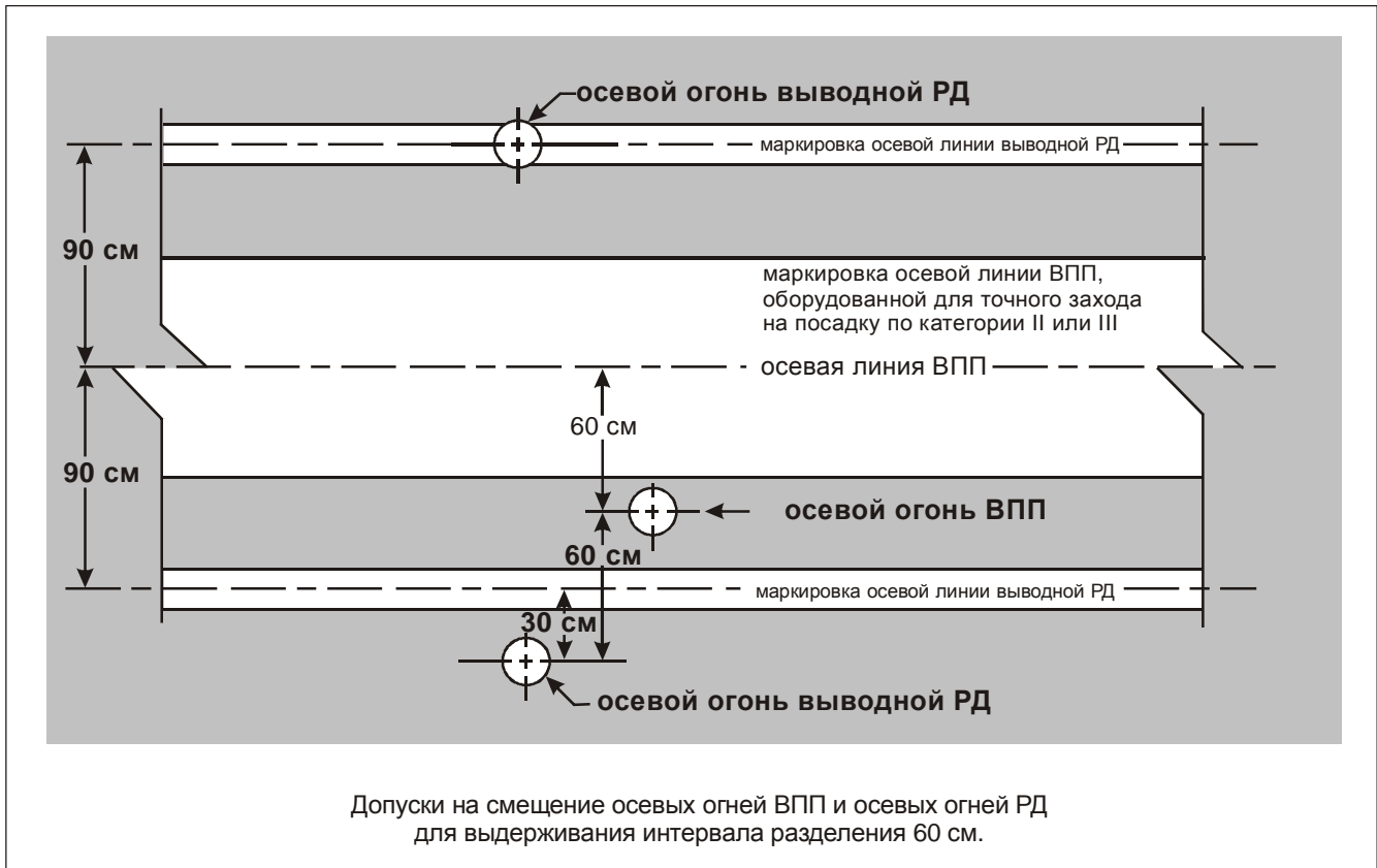
Рис. 5-26. Смещенные осевые огни ВПП и РД
