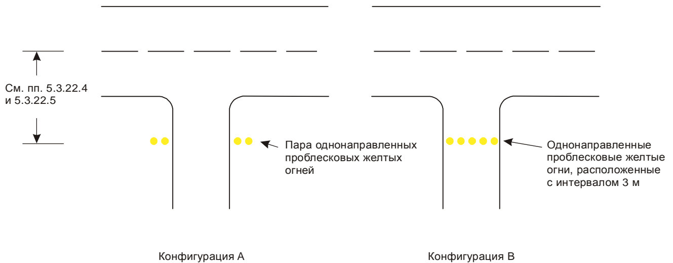
Рис. 5-28. Огни защиты ВПП
