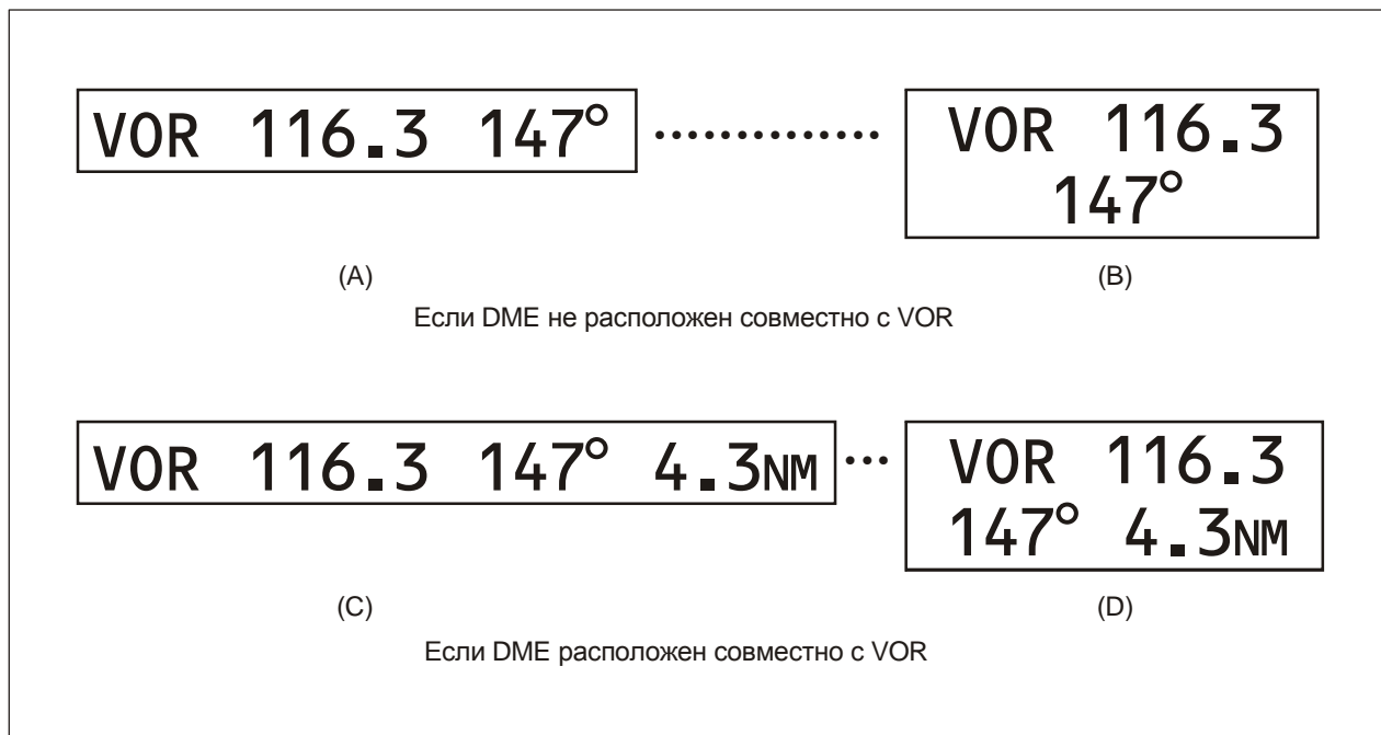
Рис. 5-32. Знак аэродромного пункта проверки VOR
