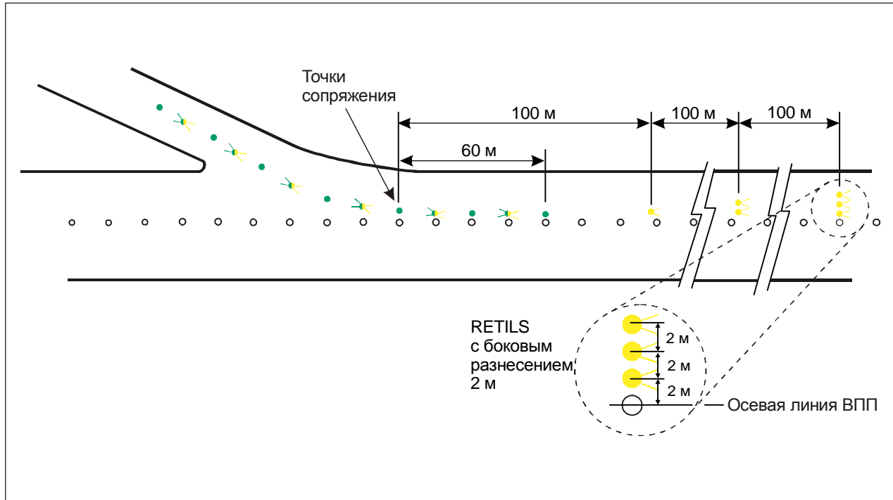
Рис. 5-24. Огни указателя скоростной выводной РД (RETILS)
