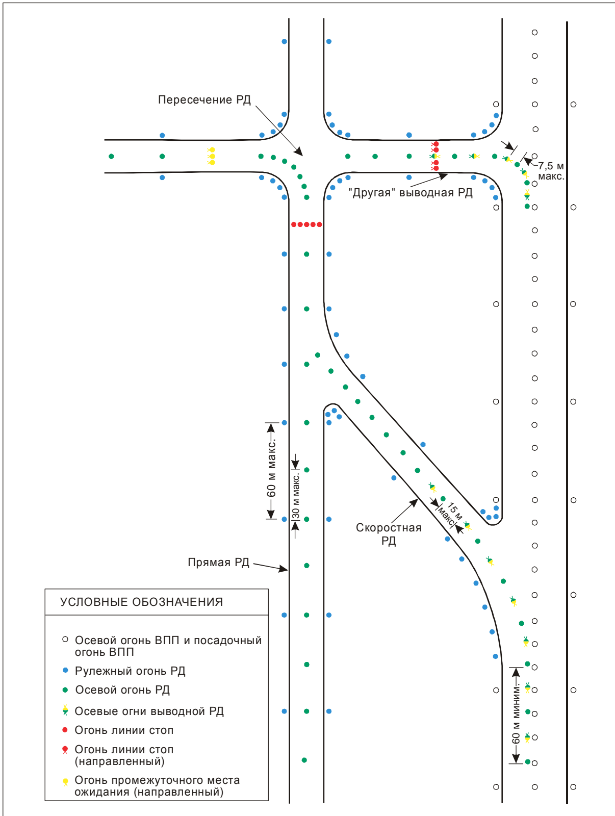
Рис. 5-25. Светосигнальная система РД
