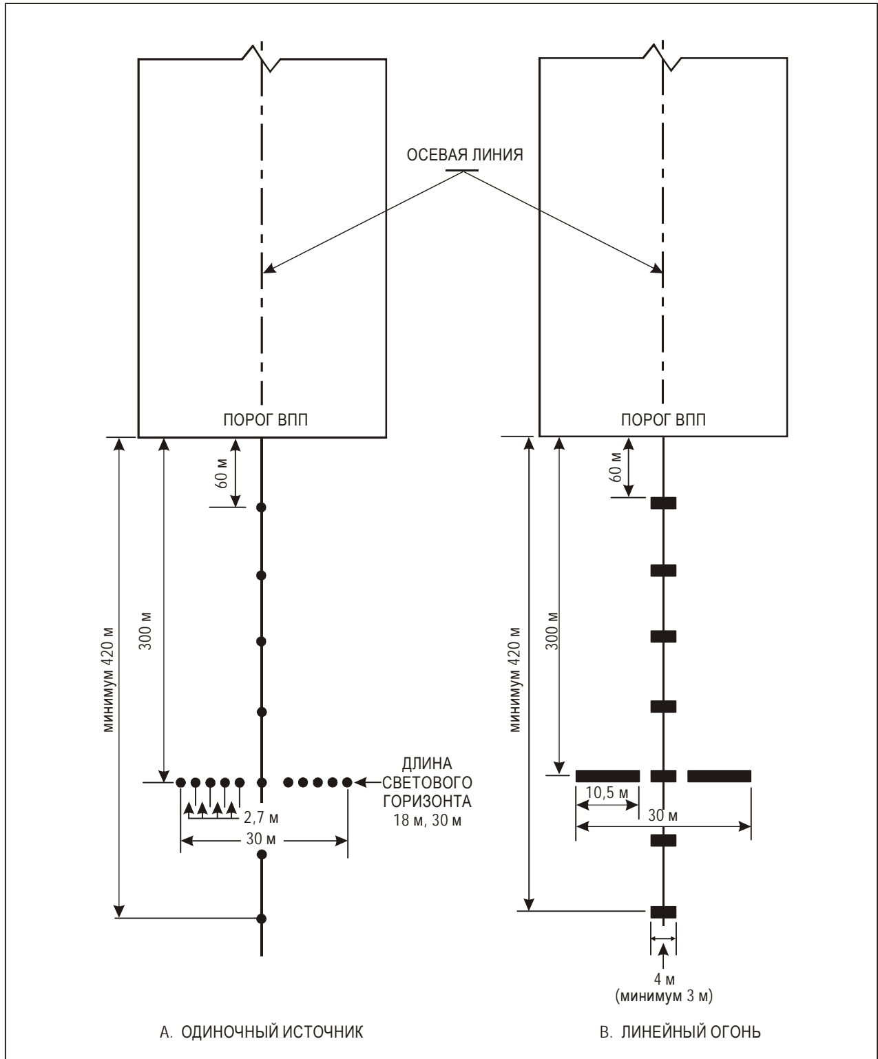
Рис. А-6. Простые системы огней приближения
