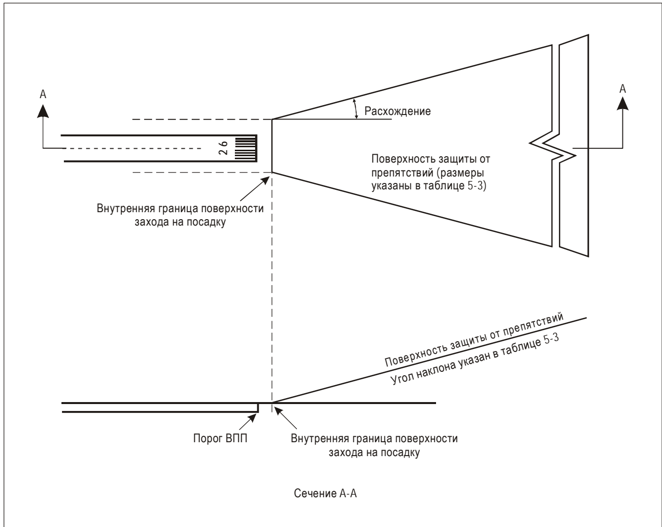
Рис. 5-21. Поверхность защиты от препятствий для систем визуальной индикации глissады
