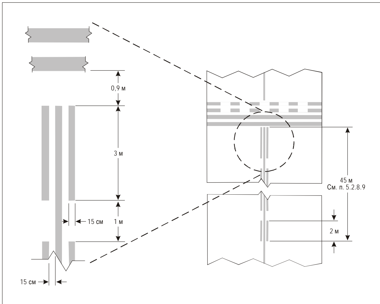
Рис. 5-7. Улучшенная маркировка осевой линии РД
