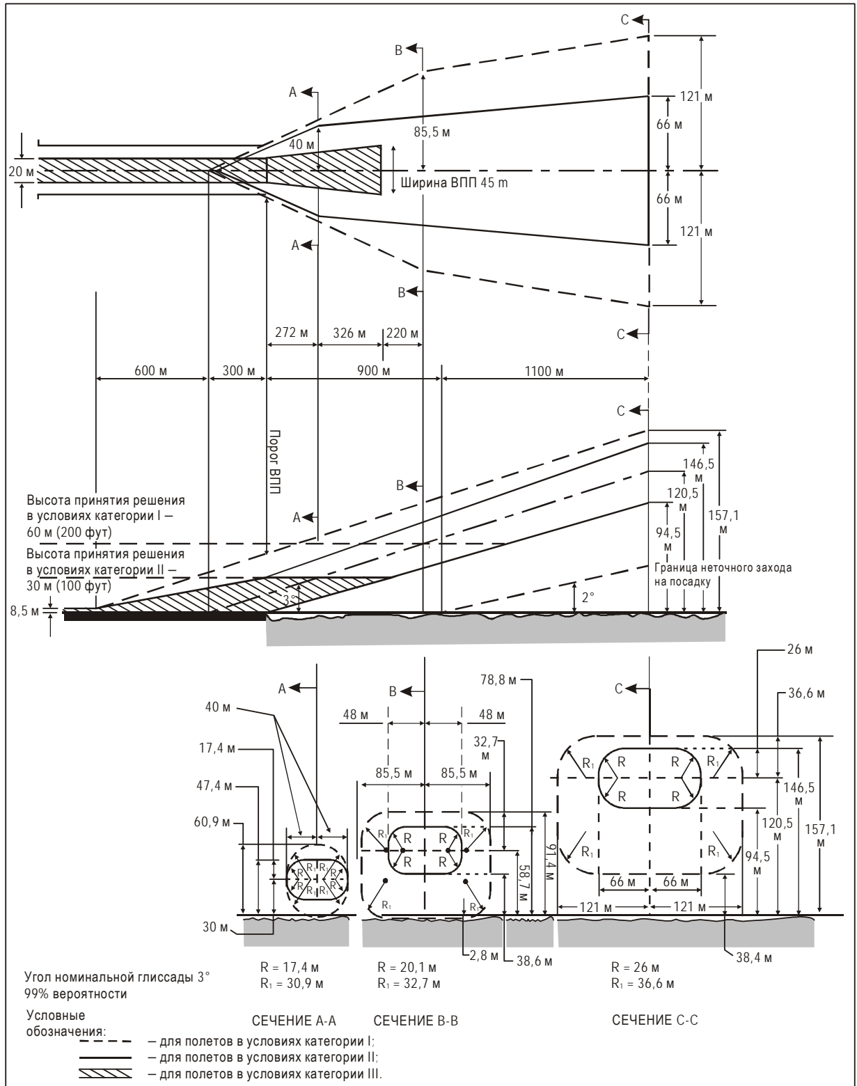
Рис. А-5. Диапазоны траектории полета, которым пользуются при проектировании светосигнальных средств для условий категории I, II и III
