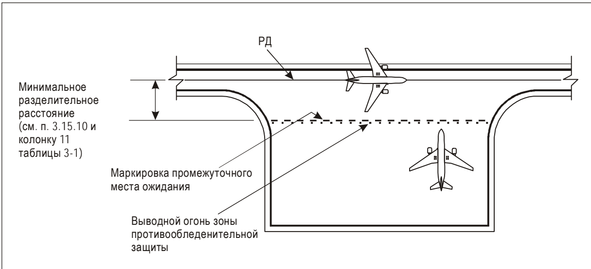
Рис. 5-27. Типичная удаленная зона противообледенительной защиты
