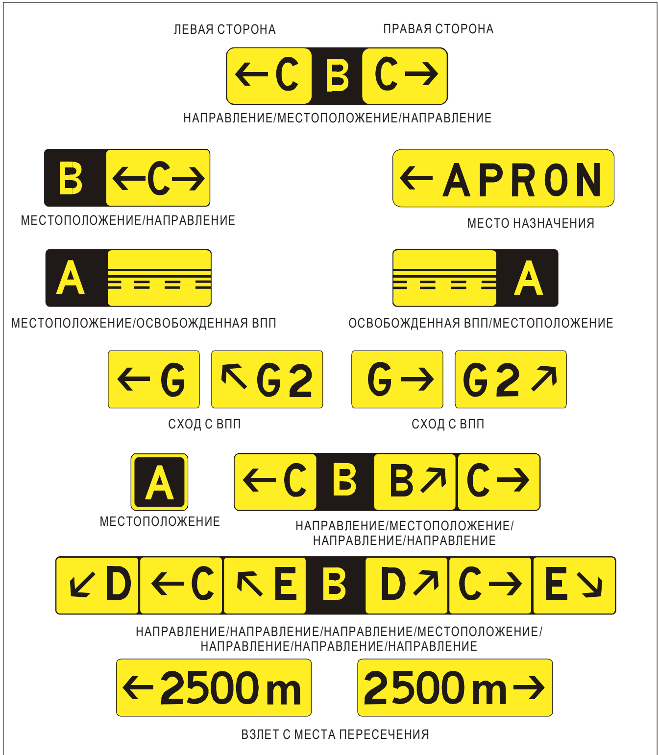
Рис. 5-30. Указательные знаки
