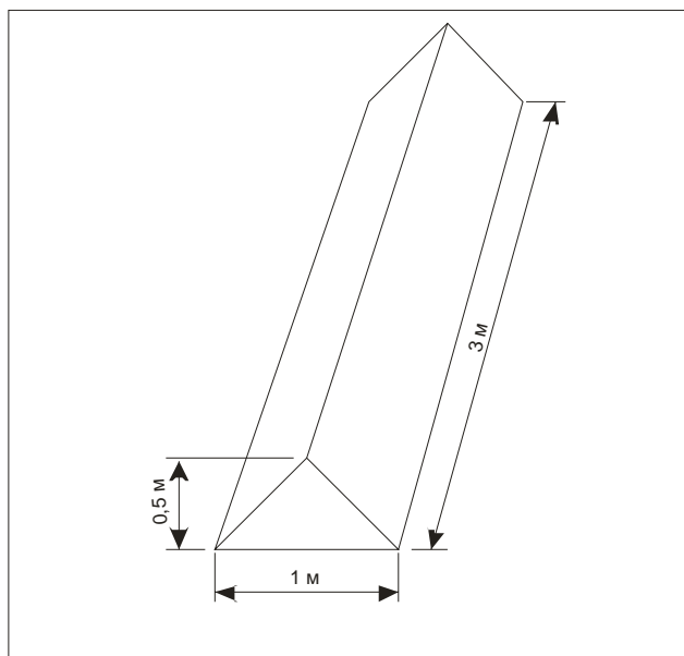
Рис. 5-33. Пограничный маркер
