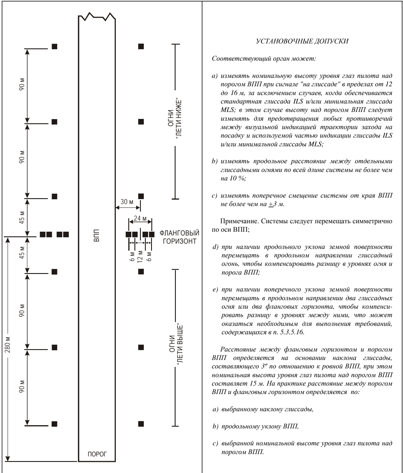
Рис. 5-17. Местоположение глиссадных огней системы T-VASIS
