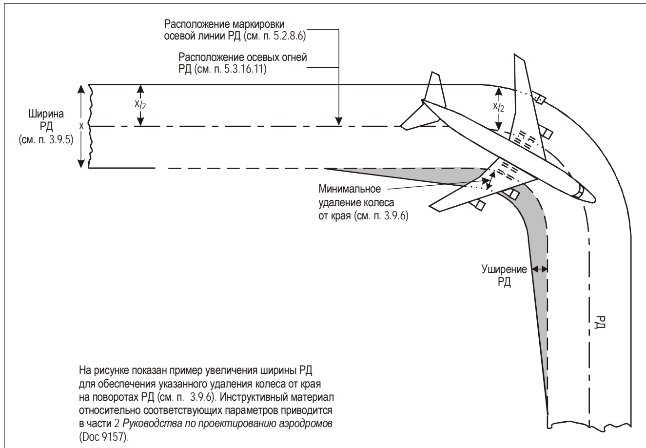
Рис. 3-2. Поворот РД
